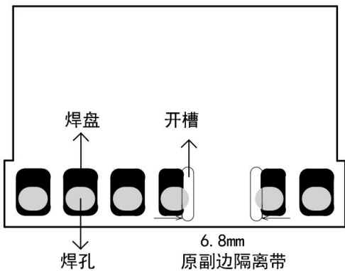
LS05-13BxxR3-F 系列推荐焊盘
