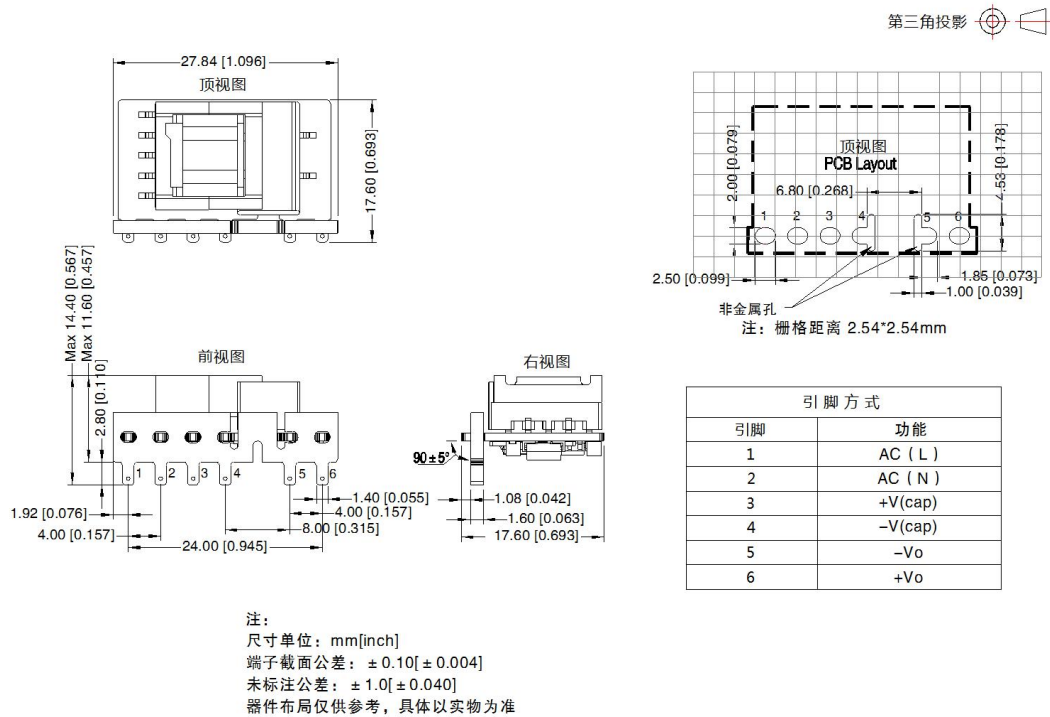
LS05-13BxxR3-F 系列推荐焊盘
