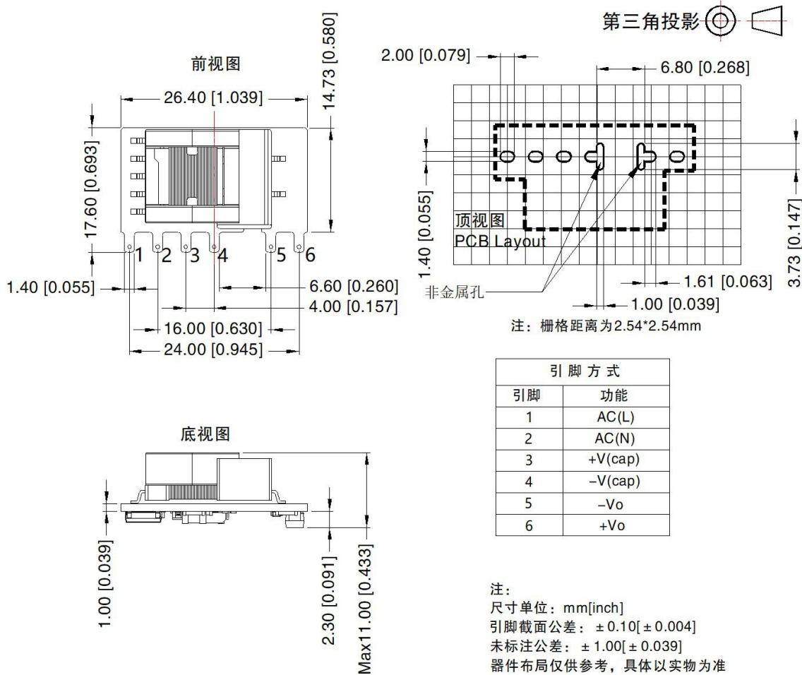
LS05-13BxxR3 系列外观尺寸图
